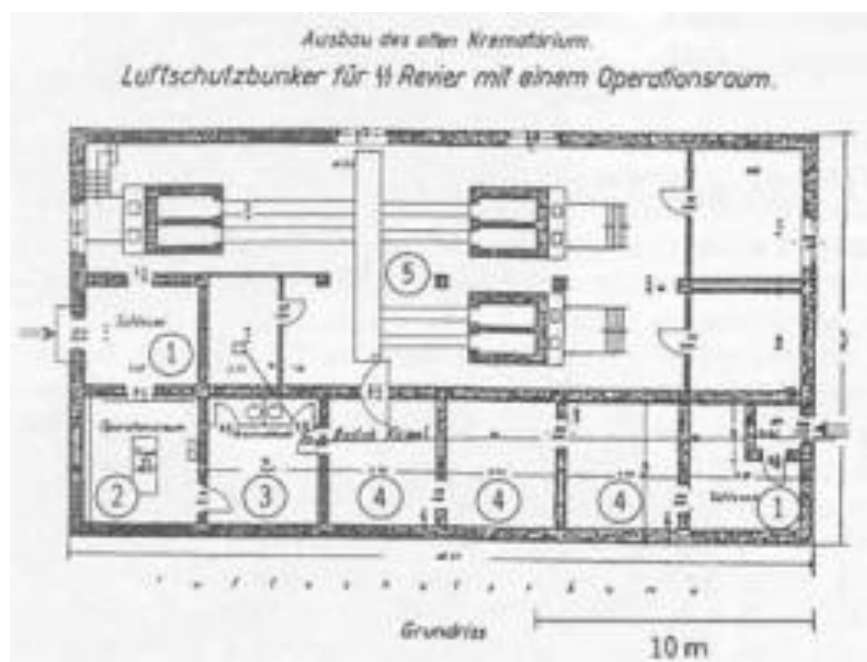
Půdorys krematoria I v Osvětimi I po přestavbě na letecký kryt provedené v roce 1944.
